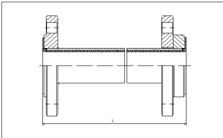
ОСНОВНИ РАЗМЕРИ (мм)
